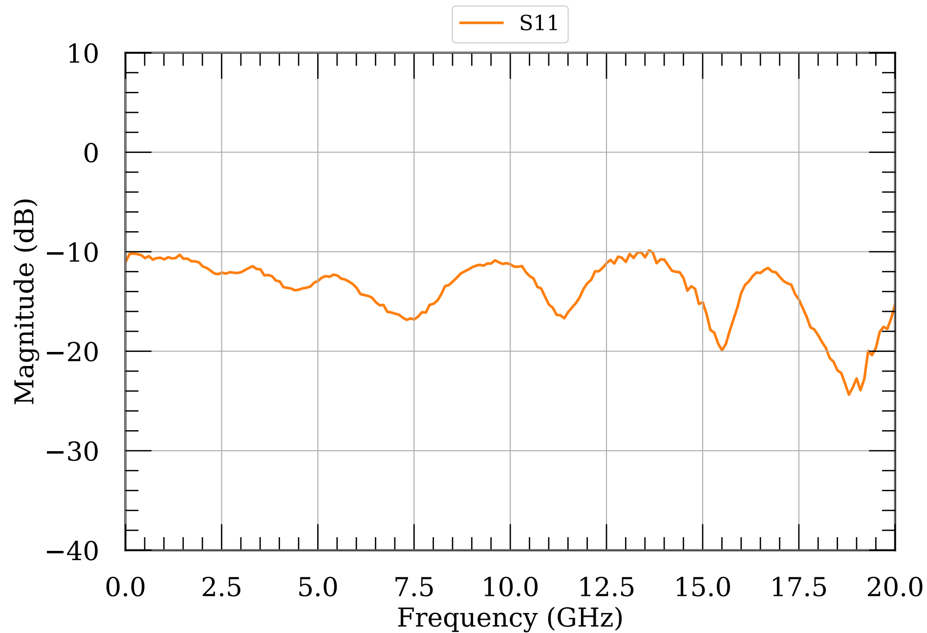
LNA S-params module036
